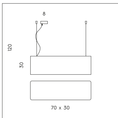
SP 7/501 2 x max 77W E27 CE IP20
