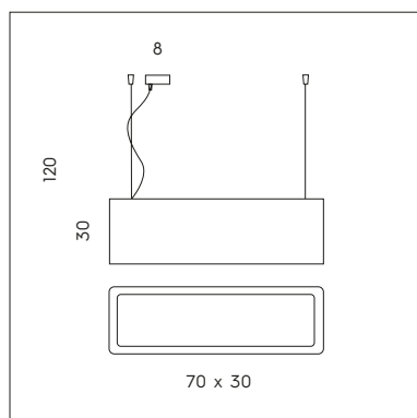
SP 7/501-L 2 x max 77W E27 CE IP20
