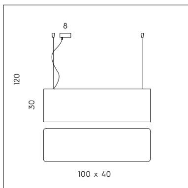
SP 8/501 3 x max 77W E27 CE IP20
