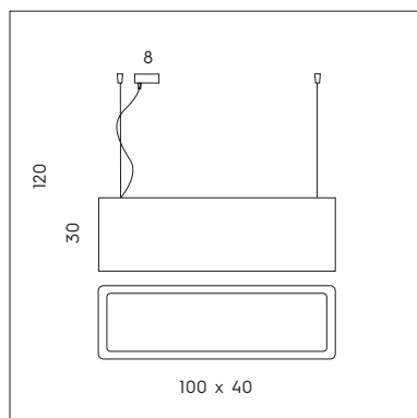
SP 8/501-L 3 x max 77W E27 CE IP20
