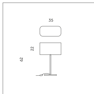
LT 1/501 1 x max 77W E27 CE IP20
